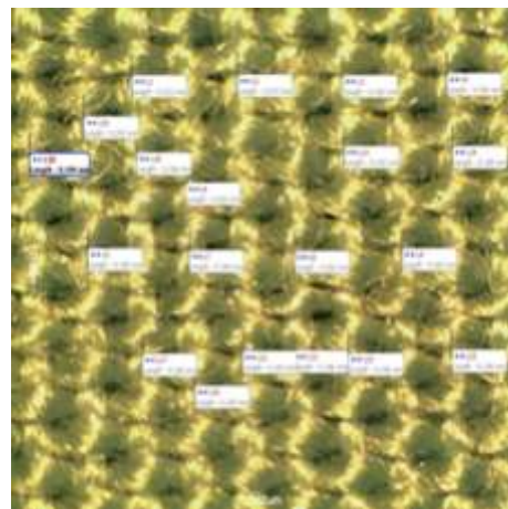
д) измерване на междуосевите разстояния между вътъчните нишки
